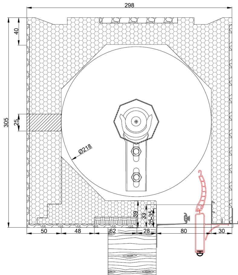
Bild 2 Schnittzeichnung (Grundsatzdetail)
