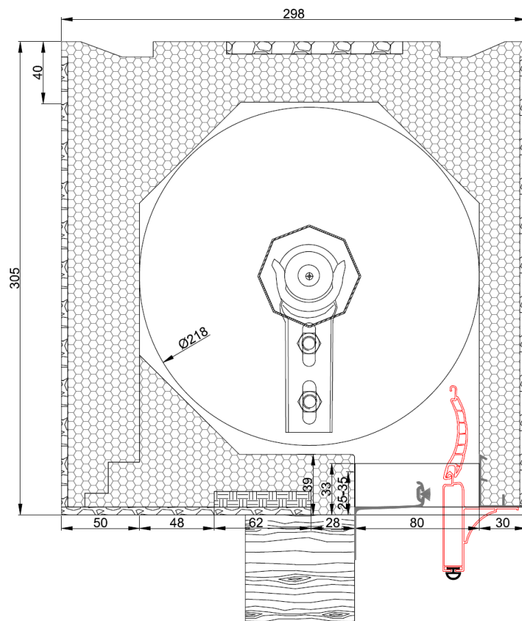
Bild 2 Schnittzeichnung (Grundsatzdetail)
