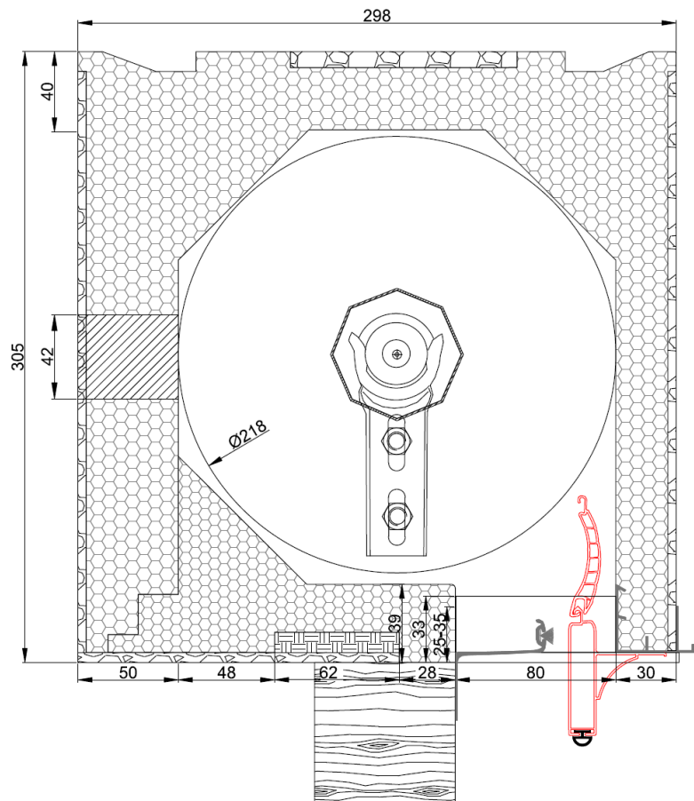
Bild 2 Schnittzeichnung (Grundsatzdetail)
